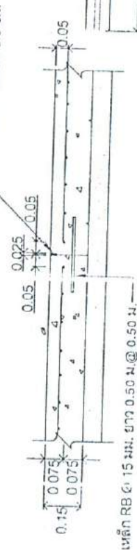
แบบขยาย LONGITUDINAL JOINT
