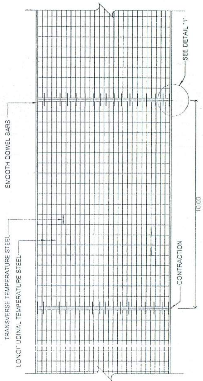
แปลนแสดงการเสริมเหล็กถนน ด.ส.ล.
