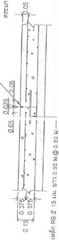
แบบขยาย CONTRACTION JOINT
